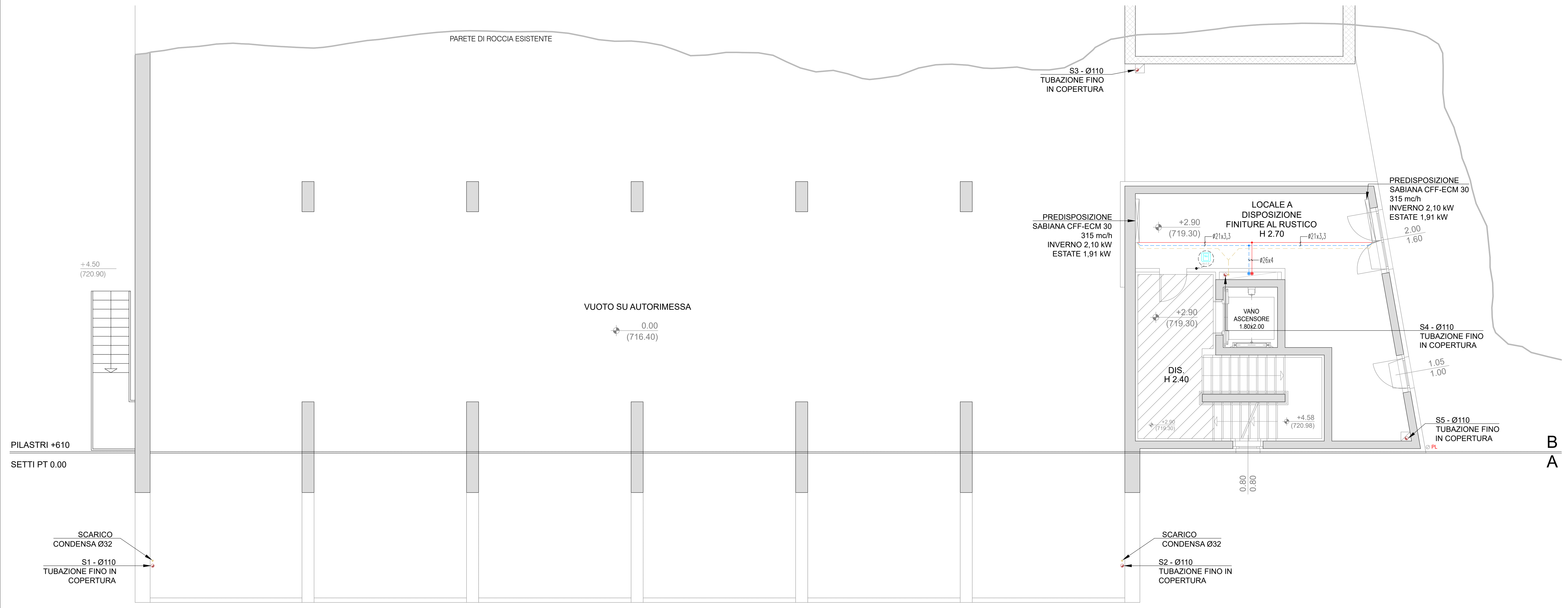
PIANTA PIANO +2,90
